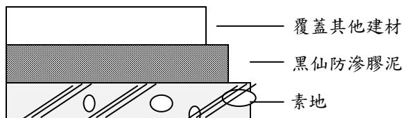
覆蓋型防滲施工圖例
